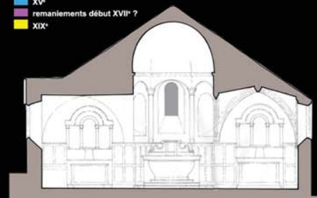
Coupe transversale - vue vers l'Est - dessin Bâtiments de France
